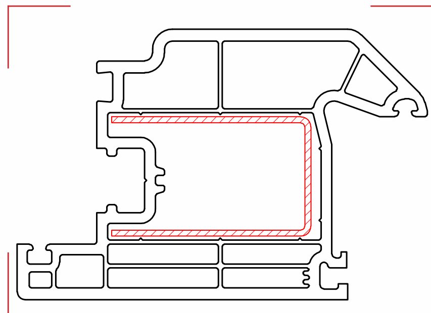
Inward Door Sash Profile
