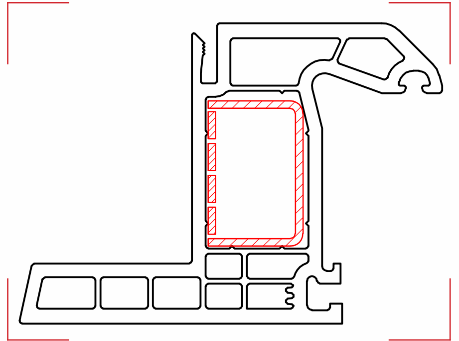
Renovation Frame Profile پروفیل قاب بازسازی
